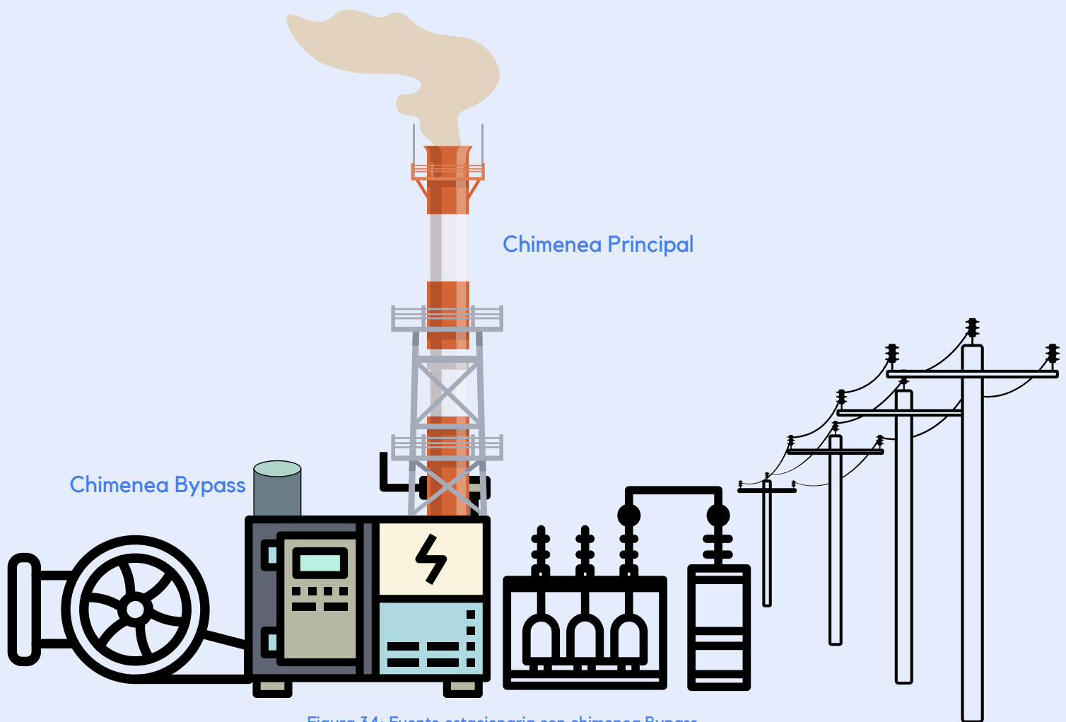
Figura 34: Fuente estacionaria con chimenea Bypass
